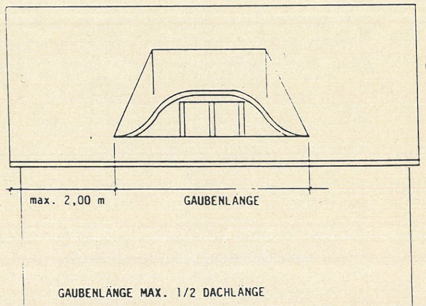
OCHSENAUGENGAUBE
